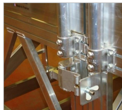
Système d'assemblage rapide des 2 parties de la plateforme
