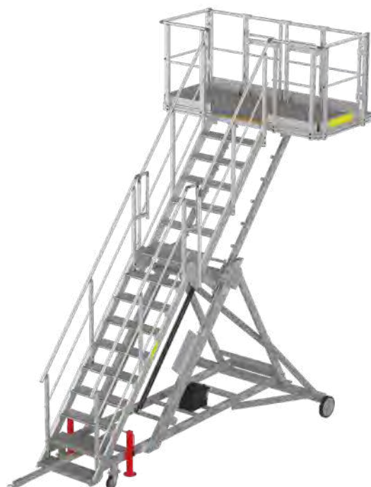
Vue 3D avant de l'escabeau
