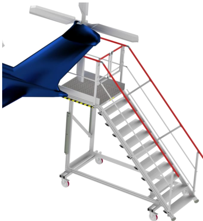
Illustration 3D escabeau en position d'utilisation
