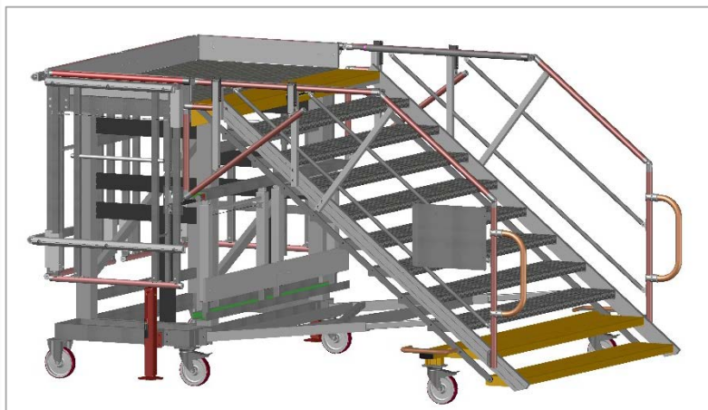
Vue 3D de l'escabeau avec garde-corps coulissants du palier en position basse
